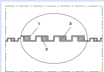
Tuyau métallique flexible d'aspiration (jusqu'à + 120 ° C)
