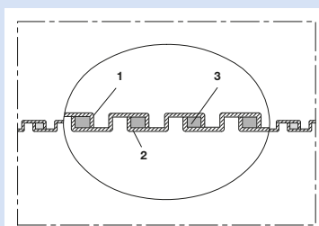
Tuyau métallique flexible d'aspiration (jusqu'à + 400 ° C)
