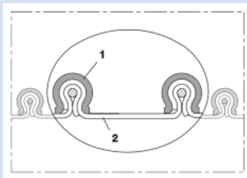
Tuyau PVC avec profilé de serrage (tuyau clippé) (jusqu'à +120°C)
