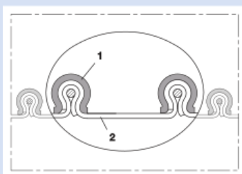
Tuyau PVC avec profilé de serrage (tuyau clippé) (jusqu'à + 110 °C)
